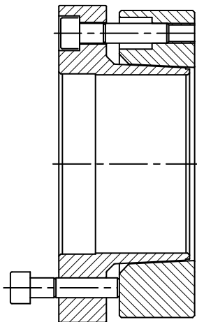
Typ 00: mit integrierter Abdrucktechnik; stirnseitig verschraubt
