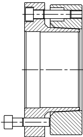
Typ 00: mit integrierter Abdrucktechnik; stirnseitig verschraubt
